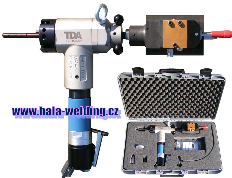
MINI TDA s pneumatickým pohonem a rychloupínáním
